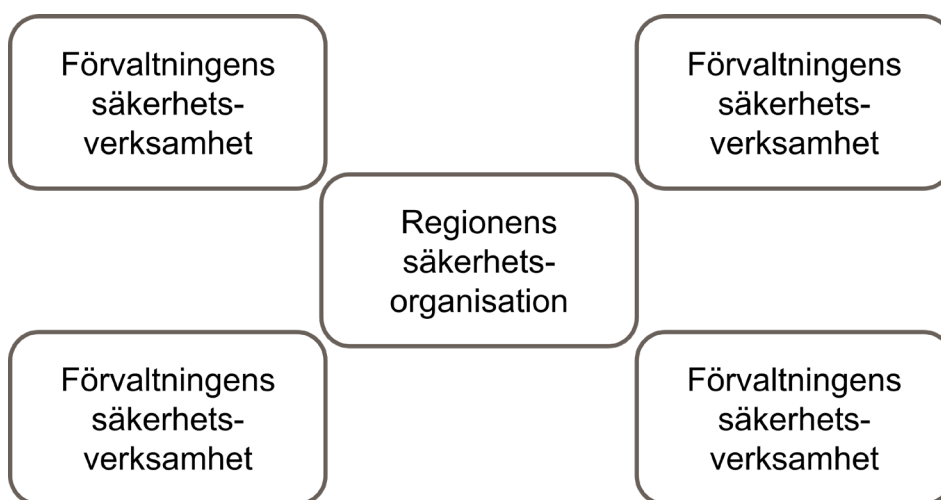
Bild 1. Decentraliserad säkerhetsorganisation
