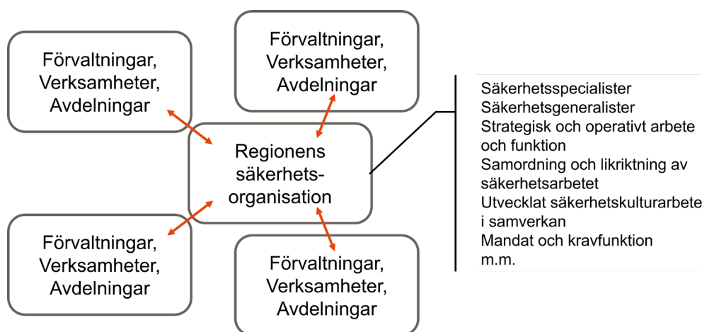
Bild 3. Centraliserad säkerhetsorganisation
